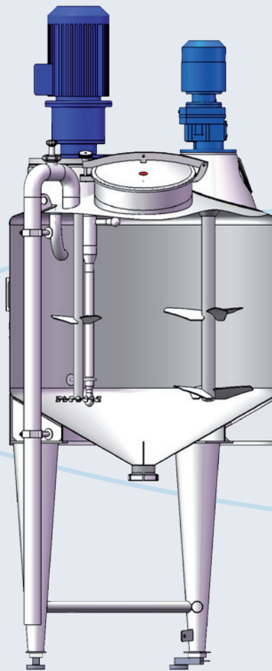
Cuve 1.000 litres atmosphérique
